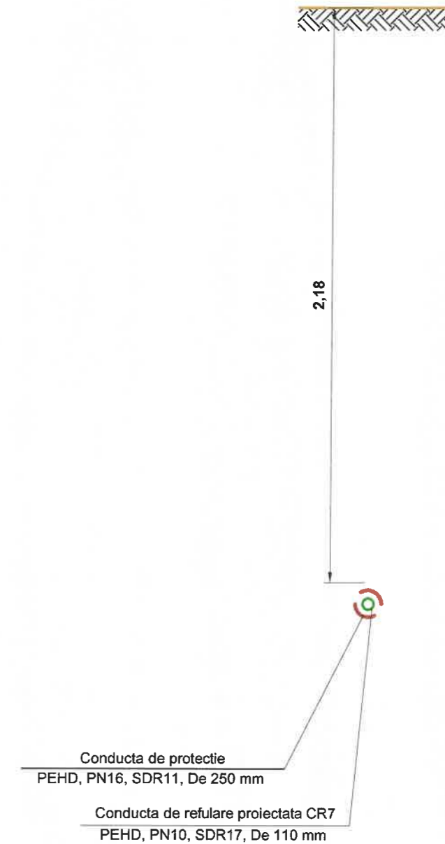
SECTIUNEA A-A Scara 1:20
